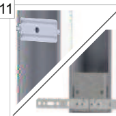
Elementy wzmacniające konstrukcję ościeżnicy z kotwami montażowymi lub bez 11. Ościeżnica 10/54,11/54 12. Ościeżnica 15/54
