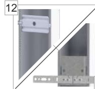
12 Elementy wzmacniające konstrukcję ościeżnicy z kotwami montażowymi lub bez 12. Ościeżnica 10/54,11/54 13. Ościeżnica 15/54
