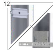
12 Elementy wzmacniające konstrukcję ościeżnicy z kotwami montażowymi lub bez 13 Ościeżnica 10/54, 11/54 12. Ościeżnica 15/54
