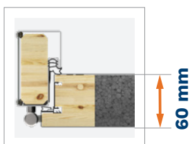
Ościeżnica DUOTHERM 60
