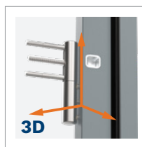
Zawiasy 3D z nasadkami, regulacja w 3 płaszczyznach
