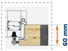
Ościeżnica ALUTHERM 60*
